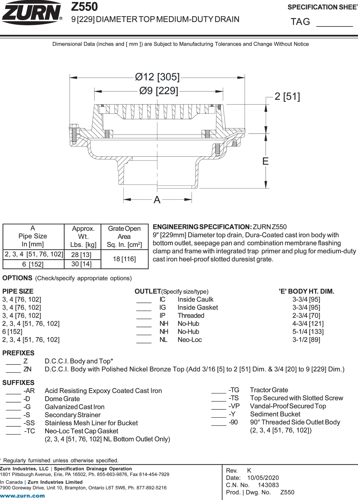
AREA DRAIN N.T.S.
