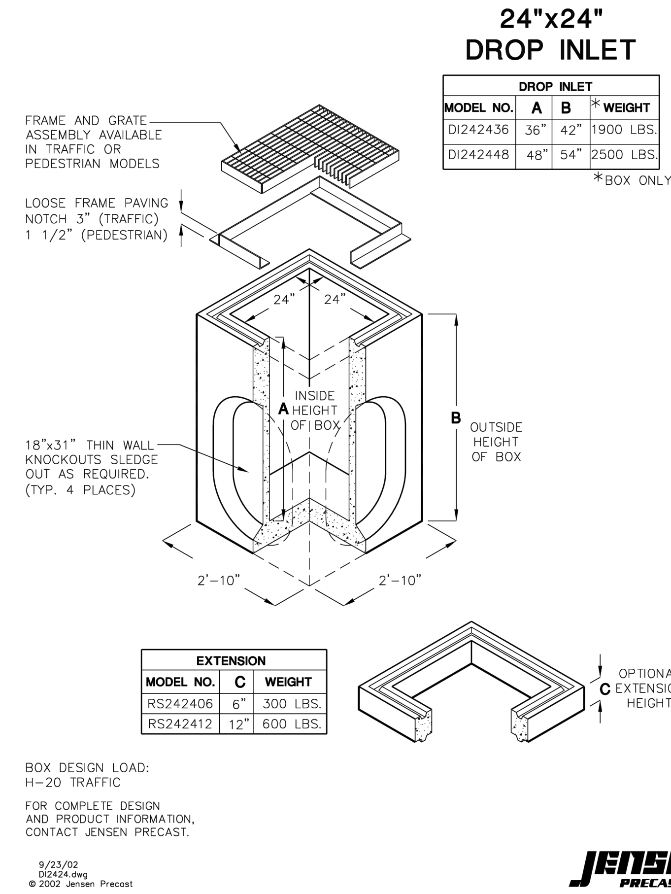
24X24 CATCH BASIN N.T.S.
