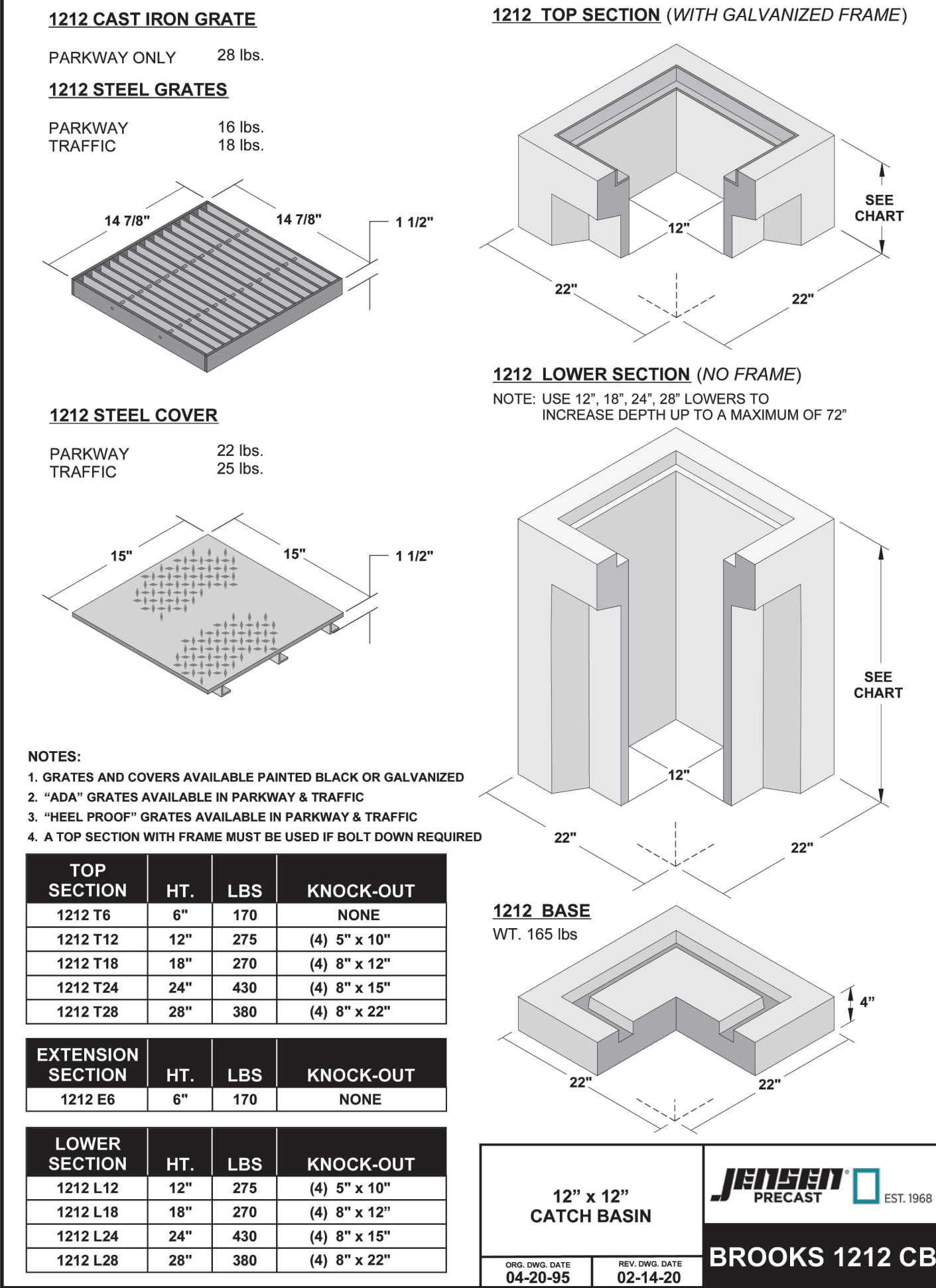
12X12 CATCH BASIN N.T.S.
