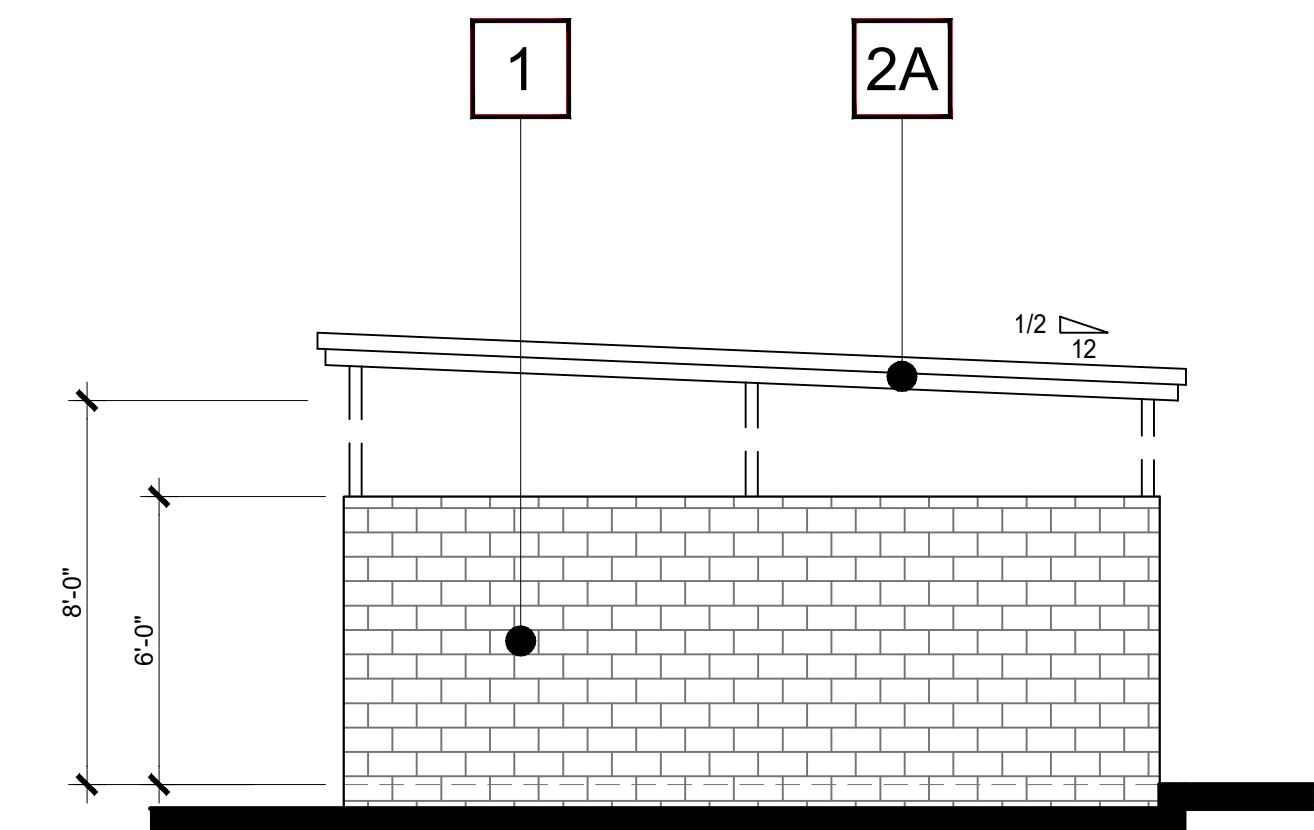
RIGHT ELEVATION 5
